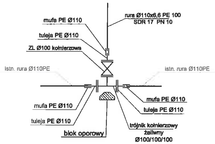
WĘZEŁ 1
