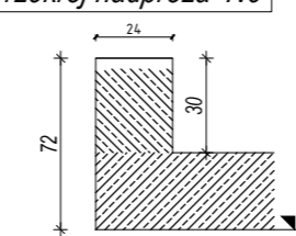
Przekrój nadproża N5 Przekrój nadproża N6
