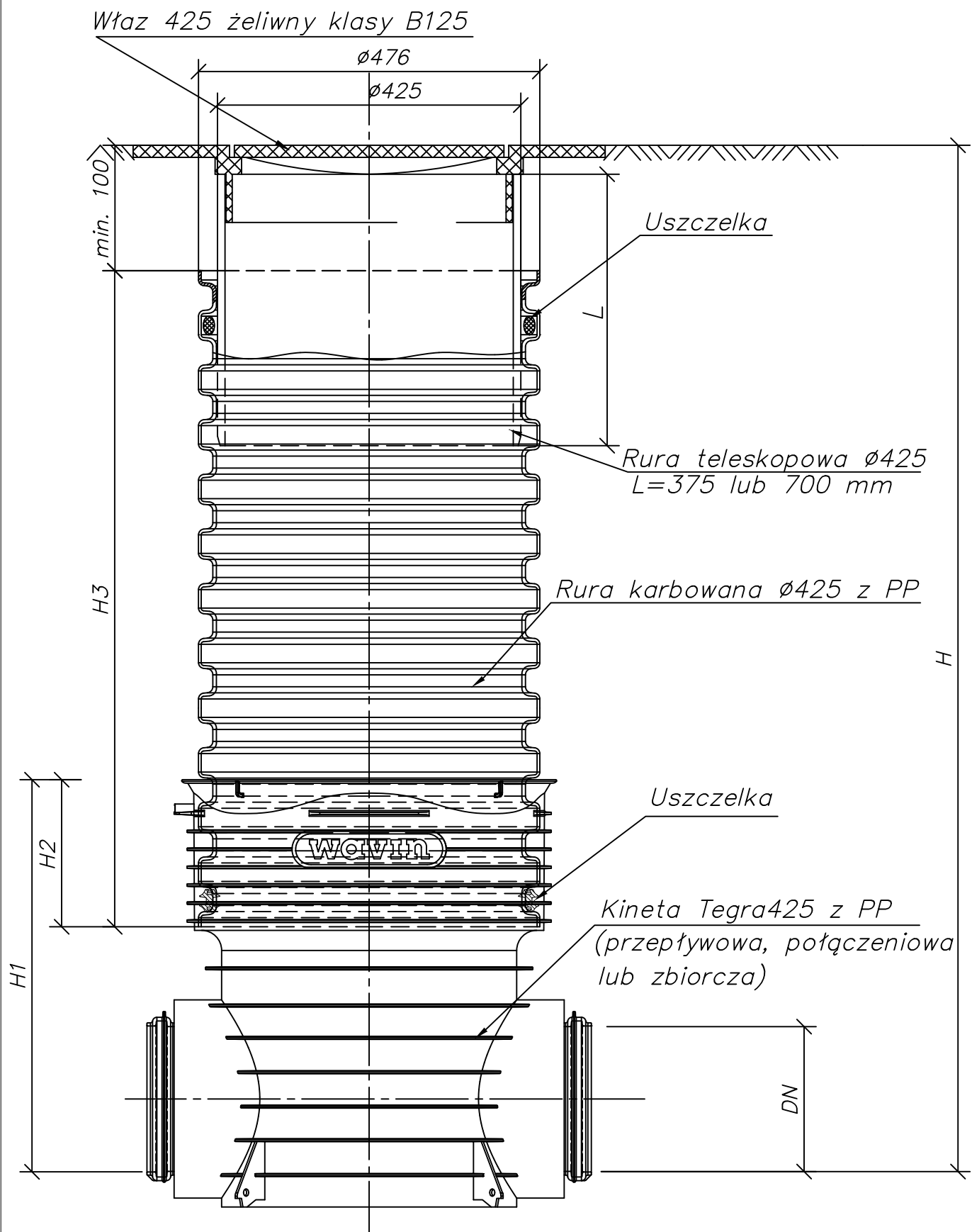
Studzienka inspekcyjna Tegra 425 z rurą teleskopową i włazem żeliwnym B
